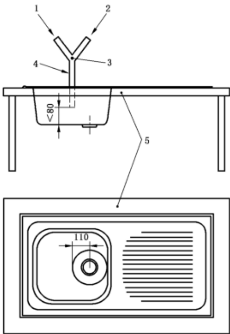
图 3 测试装置
